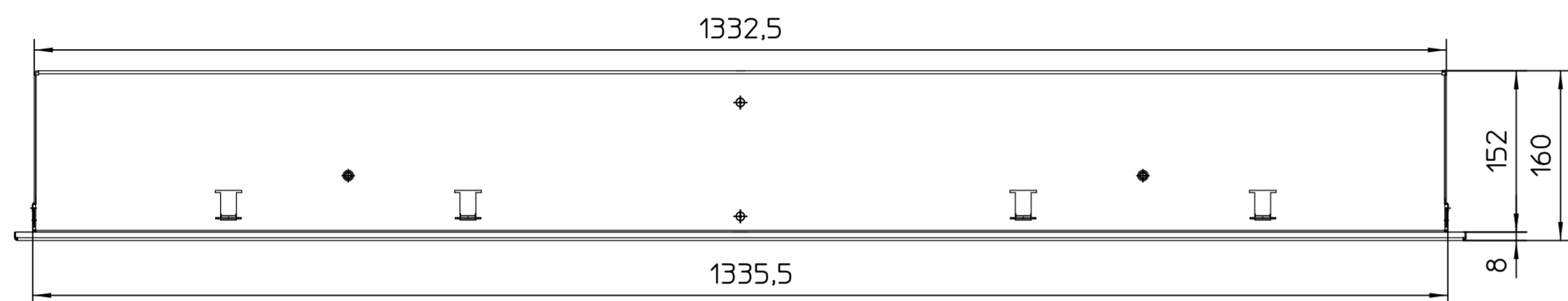
Vorderansicht 1
