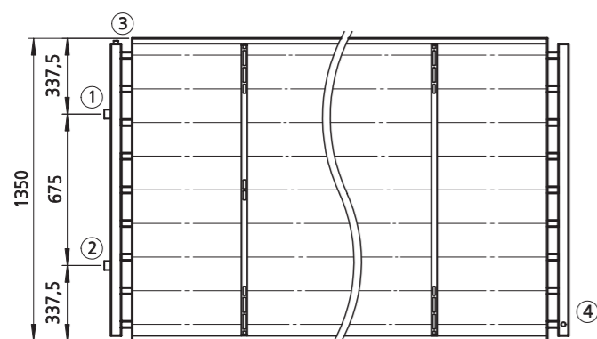
Draufsicht, einseitiger Anschluss / Top view, same-end connection
