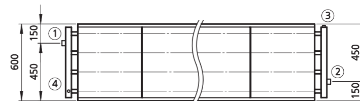
Draufsicht, wechselseitiger Anschluss / Top view, opposite-end connection
