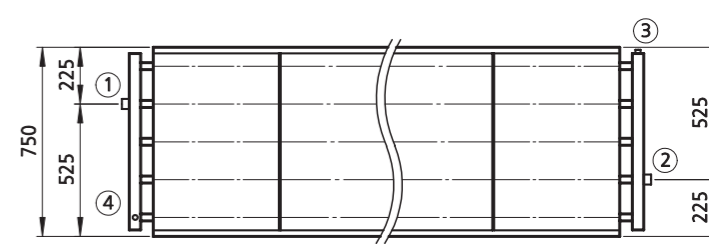
Draufsicht, wechselseitiger Anschluss / Top view, opposite-end connection
