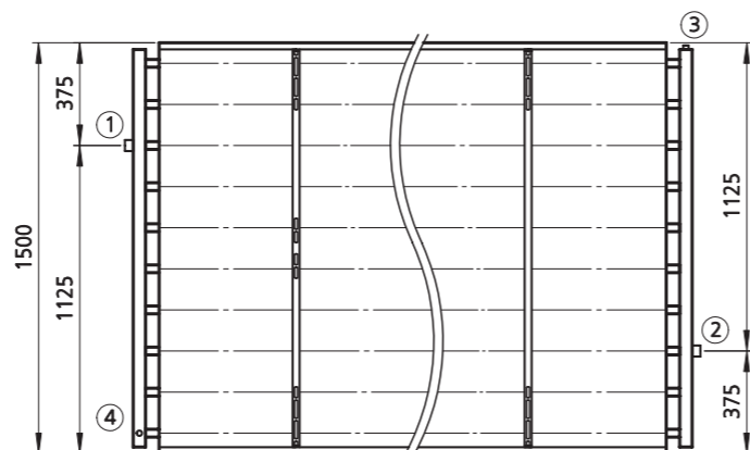
Draufsicht, wechselseitiger Anschluss / Top view, opposite-end connection
