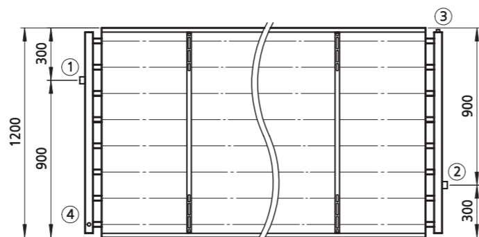
Draufsicht, wechselseitiger Anschluss / Top view, opposite-end connection
