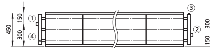
Draufsicht, wechselseitiger Anschluss / Top view, opposite-end connection
