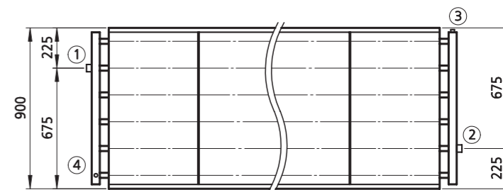
Draufsicht, wechselseitiger Anschluss / Top view, opposite-end connection
