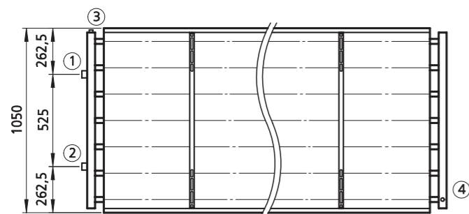
Draufsicht, einseitiger Anschluss / Top view, same-end connection
