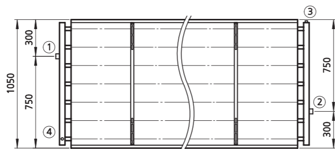
Draufsicht, wechselseitiger Anschluss / Top view, opposite-end connection
