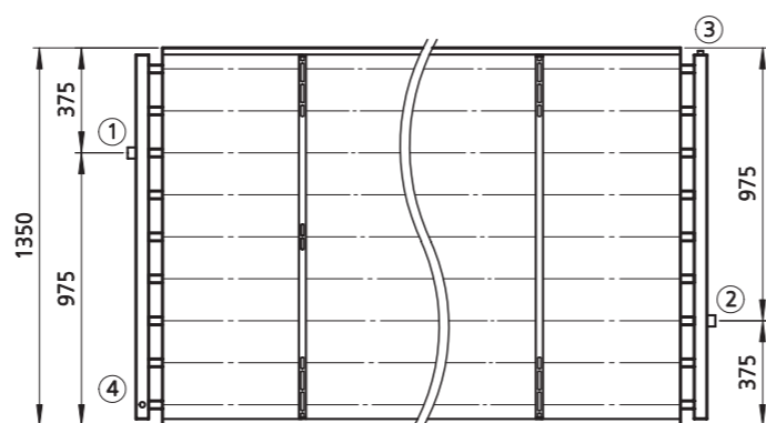
Draufsicht, wechselseitiger Anschluss / Top view, opposite-end connection
