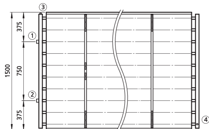
Draufsicht, einseitiger Anschluss / Top view, same-end connection
