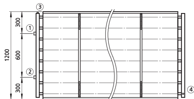
Draufsicht, einseitiger Anschluss / Top view, same-end connection
