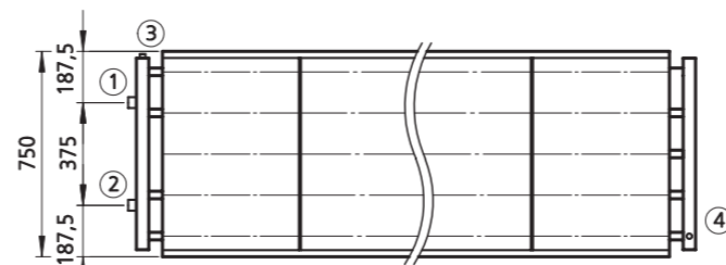
Draufsicht, einseitiger Anschluss / Top view, same-end connection
