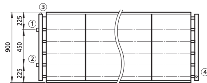
Draufsicht, einseitiger Anschluss / Top view, same-end connection
