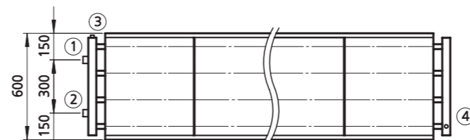
Draufsicht, einseitiger Anschluss / Top view, same-end connection
