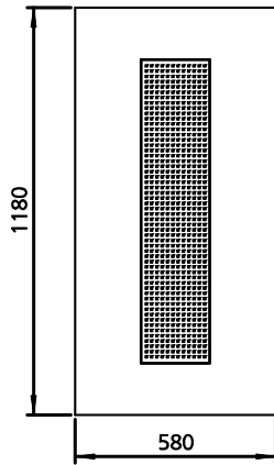
Vorderansicht
