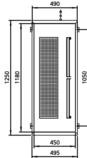
Vorderansicht
