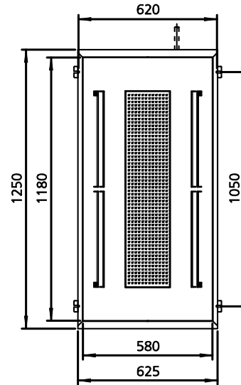
Vorderansicht
