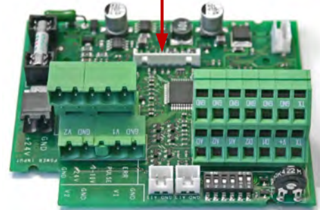
Steuerplatine
