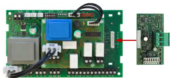
Steuerplatine
