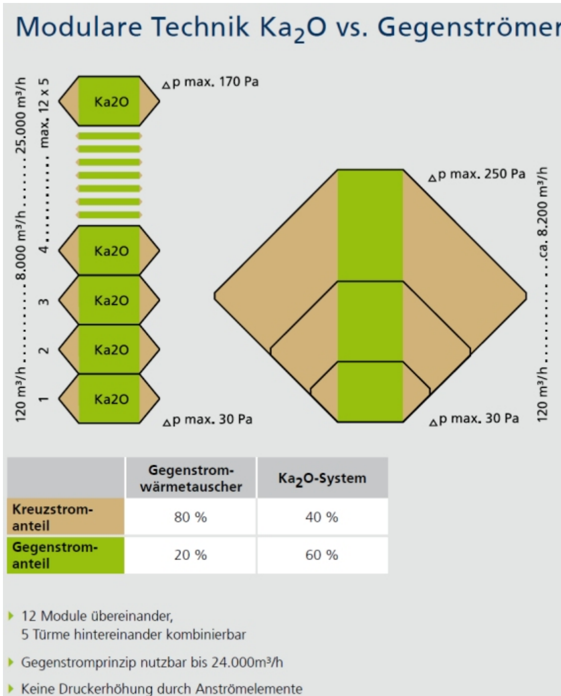
Abbildung 2: Vergleich der Modultechnik der Ka2O-Gegenstromwärmeübertrager mit einem zentralen Gegenstromwärmeübertrager
