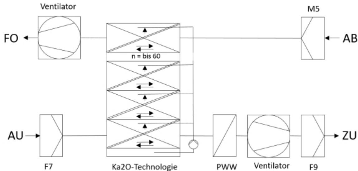
Abbildung 3: RLT-Gerät mit Ka2O-Technologie, Abluftdirektbefuchtung mit Umlaufwasser und Gegenstrom-Wärmeübertrager
